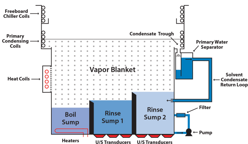
3-Sump Vapor Degreaser
